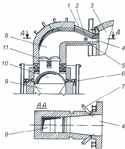
Рис. 16. Шахтная горелка с боковым подводом топлива:
