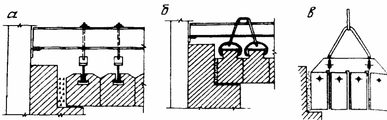
Рис. 8. Устройство подвесных сводов из фасонных кирпичей (а, б) и кирпичей с отверстиями (е)
