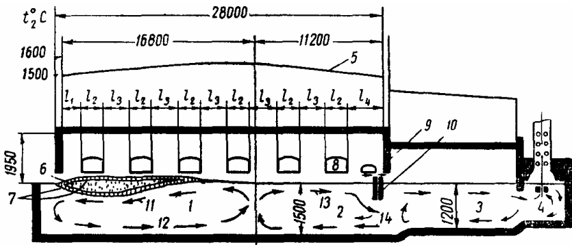
Рис. 1. Схема получения стекла в регенеративной ванной печи: 1 – зона варки; 2 – зона осветления (гомогенизации); 3 – зона студки; 4 – зона выработки листового стекла; 5 – температурная кривая; 6 – слой шихты; 7 – слой расплава; 8 – воздушные влеты горелок; 9 – разделительный экран; 10 – заградительный порог в стекломассе; 11 – ветвь потока стекломассы в варочной зоне, верхняя; 12 – то же, нижняя; 13 – ветвь потока стекломассы в зоне осветления, верхняя; 14 – то же, обратная
