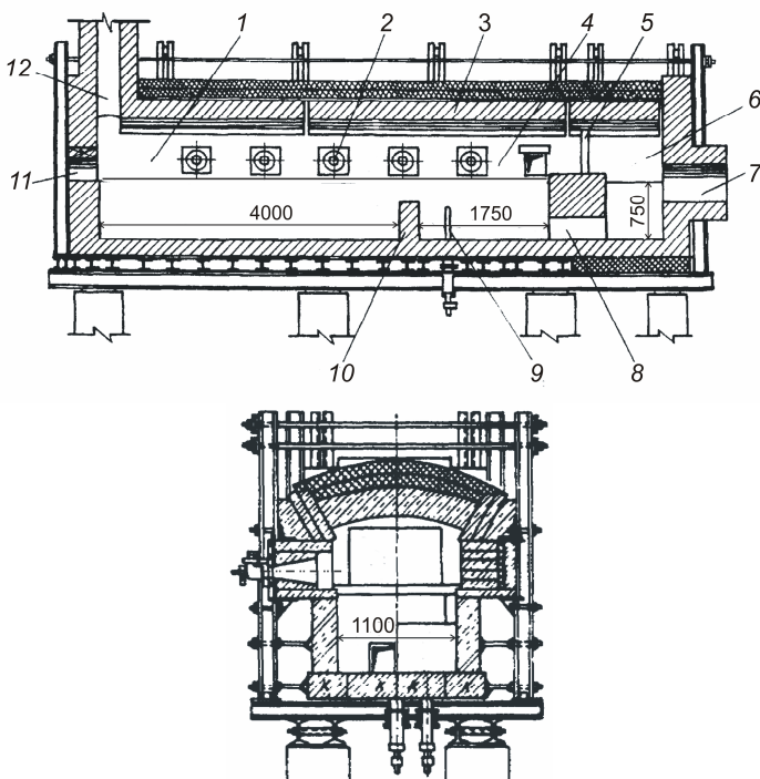
Рис. 6. Продольный и поперечный разрезы печи прямого нагрева: 1 – зона варки; 2 – горелки; 3 – свод печи; 4 – зона освещения; 5 – разделительный экран; 6 – студочная часть; 7 – выработочный канал; 8 – проток; 9 – электрод; 10 – порог; 11 – загрузочное отверстие; 12 – газоотводящий канал
