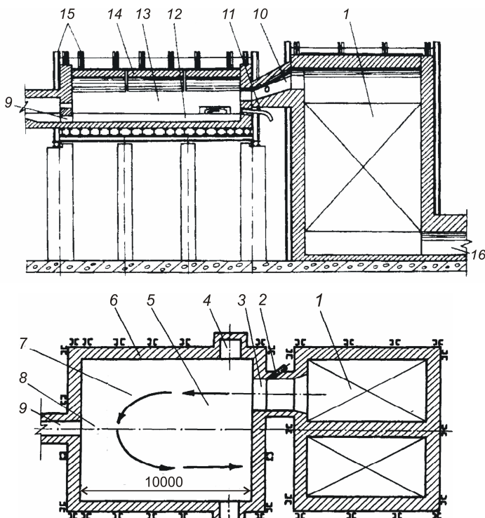
Рис. 4. Ванная регенеративная печь с подковообразным пламенем: 1 – насадка регенератора; 2 – боковая подача топлива; 3 – влет горелки; 4 – загрузочный карман; 5 – варочная зона; 6 – стены печи; 7 – зона освещения; 8 – зона стужки; 9 – проток; 10 – подвод воздуха; 11 – нижний подвод топлива; 12 – стекломасса в бассейне; 13 – пламенное пространство; 14 – свод печи; 15 – металлический каркас печи
