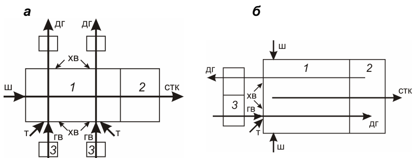
Рис. 18. Тепловые схемы стекловаренной печи с поперечным (а) и подковообразным (б) направлением пламени: 1 – варочная часть; 2 – студочная часть; 3 – регенератор; ш – шихта; стк – стекломасса; т – топливо; гв – горячий воздух; хв – холодный воздух; дг – дымовые газы
