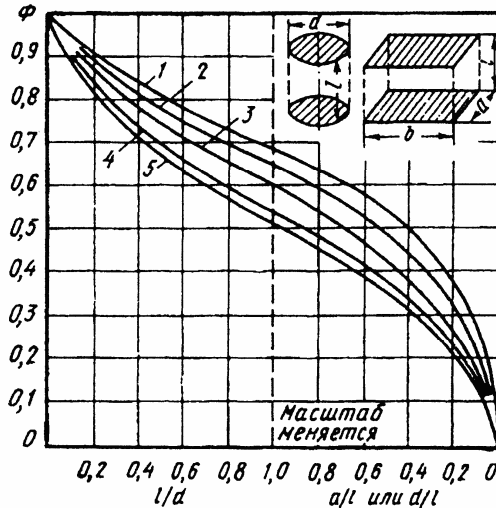
Рис 19. График, определяющий коэффициент диафрагмирования: 1 – узкая длинная полоса; 2 – прямоугольник ( a : b = 0,2 ); 3 – прямоугольник ( a : b = 0,5 ); 4 – квадрат; 5 – круг
