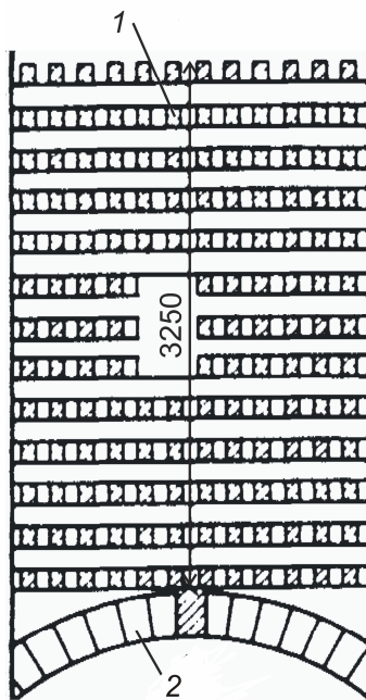
Рис. 22. Расположение насадки регенератора в газоходе: 1 – кирпичная насадка; 2 – нисующие арки
